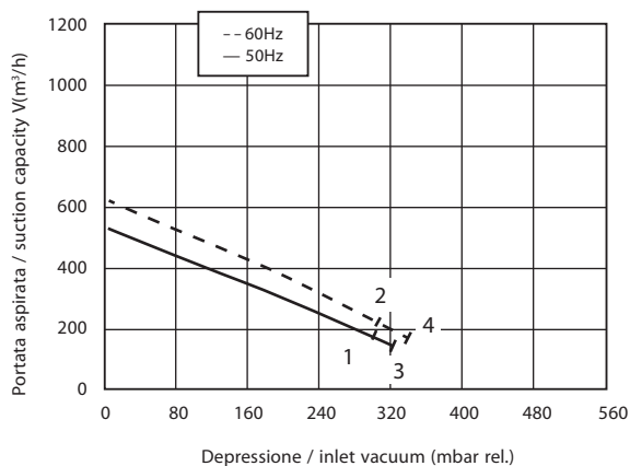
ASPIRAZIONE / EXHAUST
