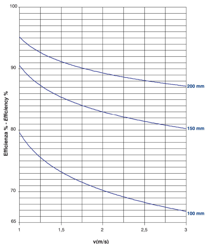
Légnedvesítési hatások a légsebesség függvényében
