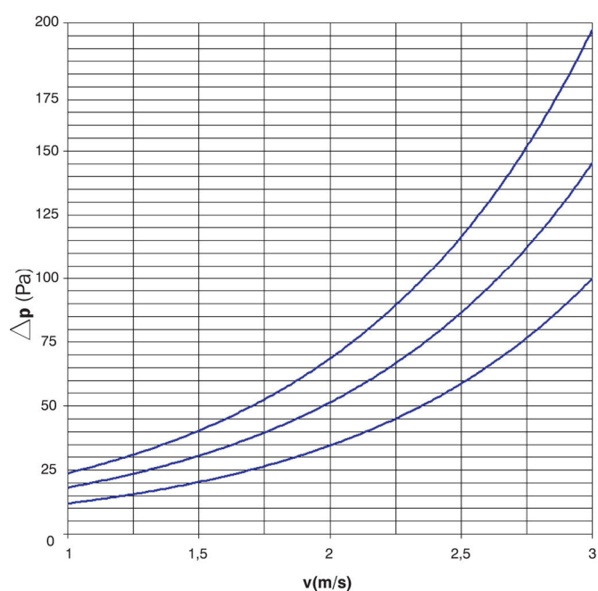
Nyomáscsökkenés a légsebesség függvényében
